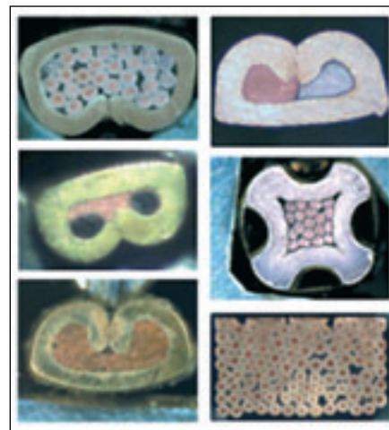
Imagini de slifuri pentru diverse sectiuni de cablu si terminale, realizate cu ajutorul SK 4000
